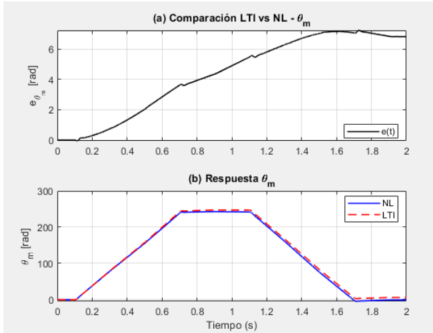
Figura 21: Comparación \theta_m para LTI y NL
