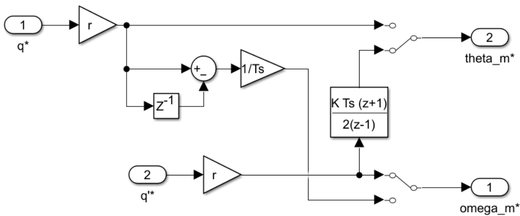
Figura 90: Set-point Discretizado
