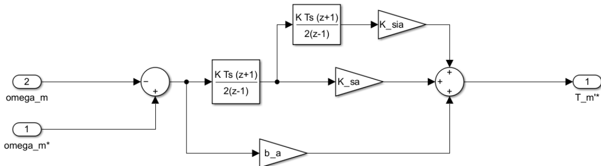
Figura 91: PID externo discretizado
